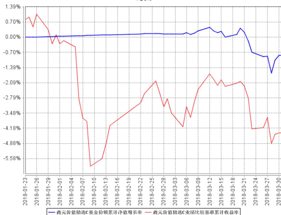
鑫元价值精选C基金份额累计净值增长率与同期业绩比较基准收益率的历史走势对比图
